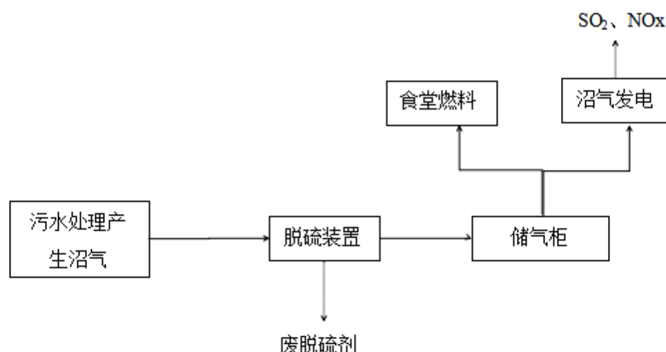
图 3.5-5 沼气工程工艺流程及产污环节图
