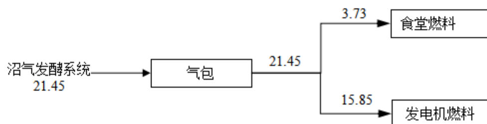
图 3.6-3 沼气平衡图
